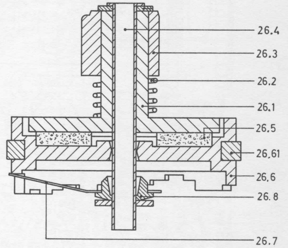
Embrayage complet (5100-090)
