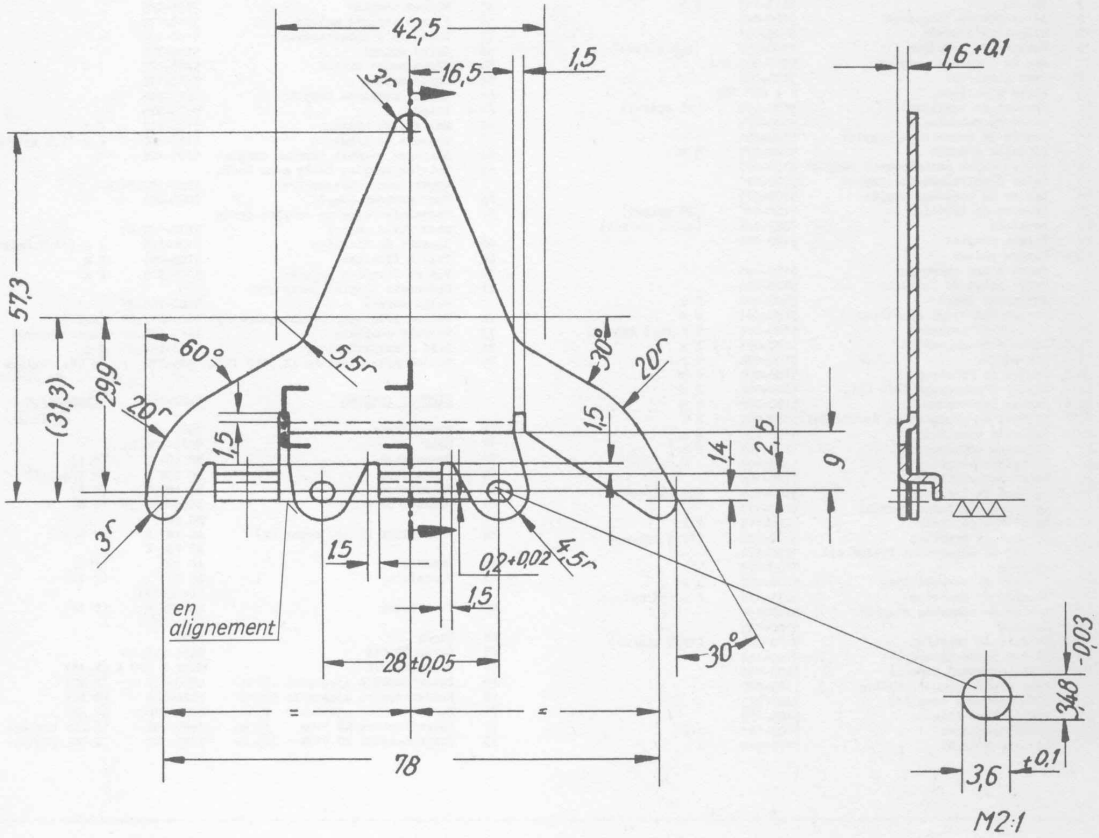
Gabarit N° 5999-069 pour le réglage des têtes
